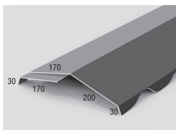
Faîtière double Doppelte First Dubbele nok Double ridge course Cumbreira doble
