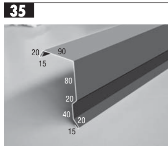
Rive extérieure Ortblech aussen Windveer buiten Outer Flashing Cenefa lateral
