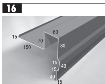
Pièce de rive Ortblech Windveer Flashing Cenefa lateral
