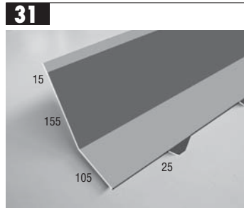
Faîtière en solin Firstzahnblech Muurnok Ridge wall connection Union mural dentada
