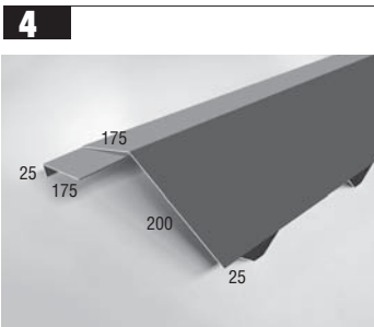
Faîtière double Doppelte First Dubbele nok Double ridge course Cumbrera doble
