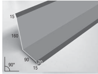
Raccord mural Maueranschluss Muuraansluiting Wall linkage Union mural
