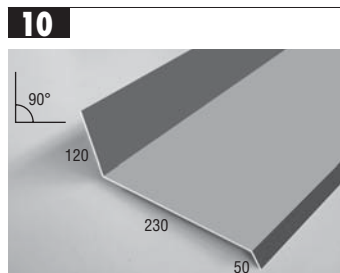
Raccord mural Maueranschluss Muuraansluiting Wall linkage Union mural
