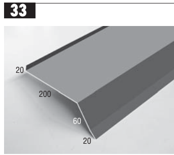
Solin de finition Traufkappe Druiplijst Eaved plate Remate del alero
