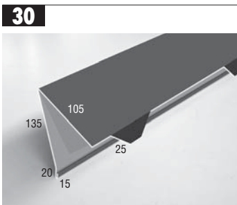
Protection murale Einhängige First Eenhangige nok Pent ridge course Protector mural en punta
