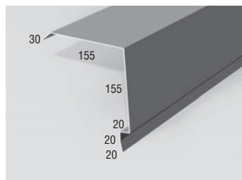
Pièce de rive Ortblech Windveer Flashing Cenefa lateral
