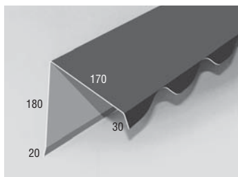
Protection murale Einhängige First Eenhängige nok Pent ridge course Protector mural en punta
