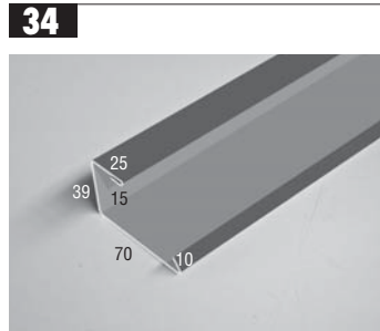
Rive intérieure Ortabschluss innen Windveer binnen Inner Flashing Cenefa interior
