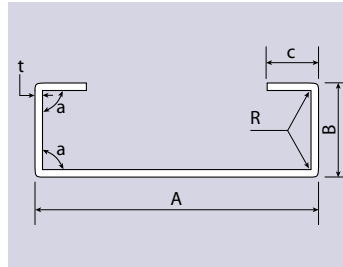
Profilé CE
