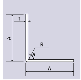
Cornière
