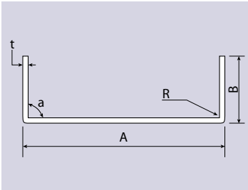
Profilé U
