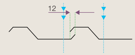
Position des fixations en plage
