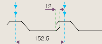
Position des fixations en sommet d'ondes
