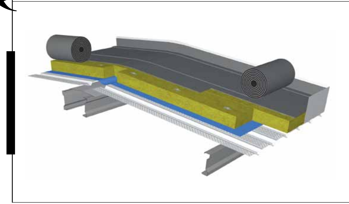
GLOBALROOF CN 1115i con estanqueidad / com impermeabilização
