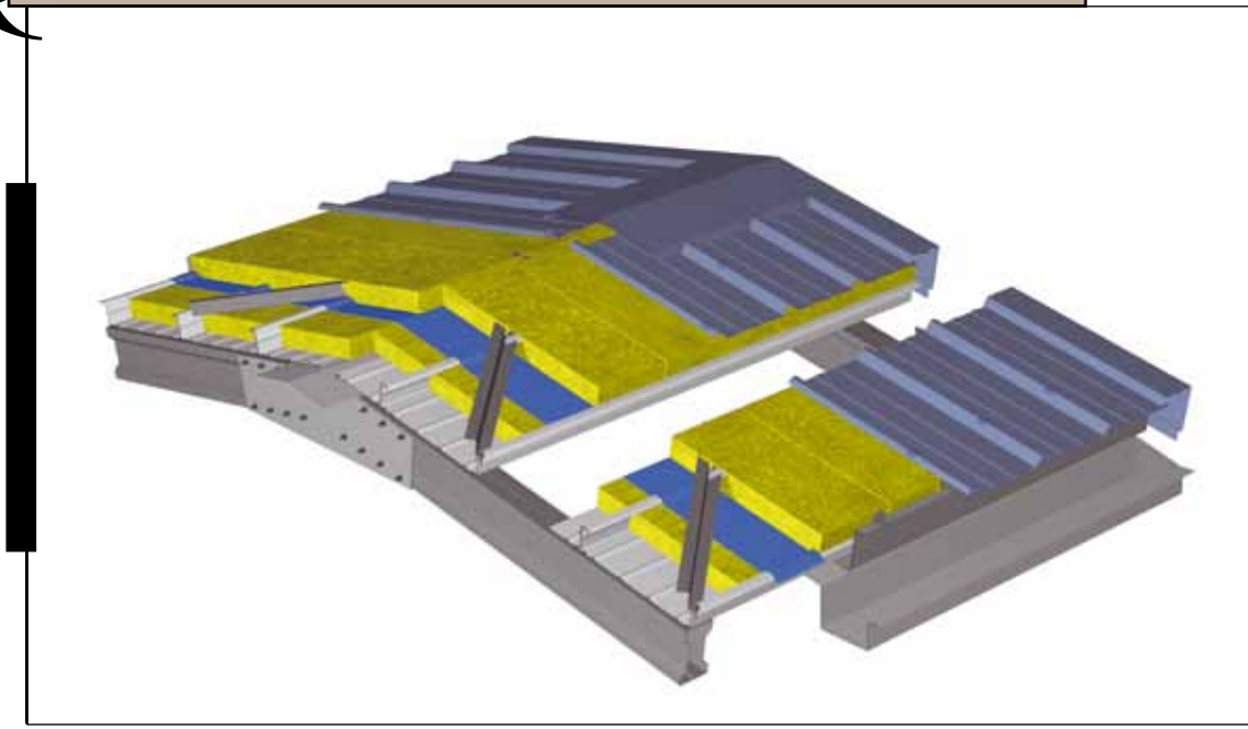
GLOBALROOF CIN 327 tramas cruzadas en cubierta / trama cruzada na cobertura
