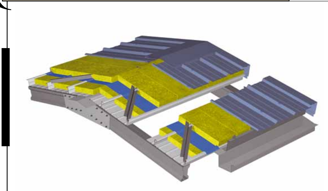
GLOBALROOF CIN 327 trames croisées en couverture / roof-covering cross-frames
