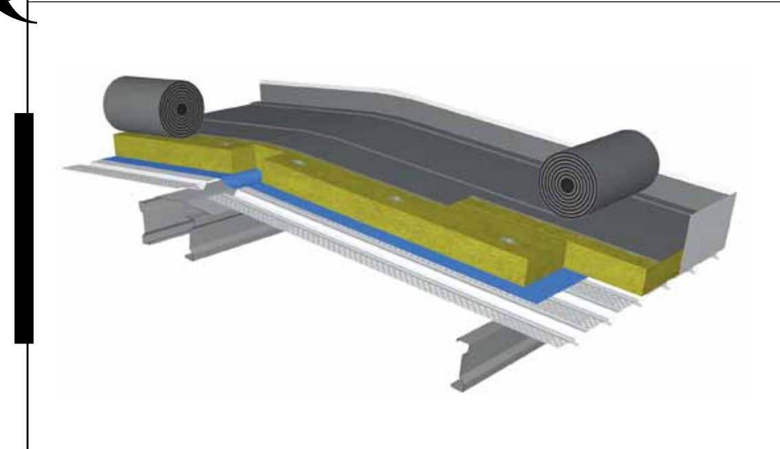
GLOBALROOF CN 1115i avec étanchéité / with sealing
