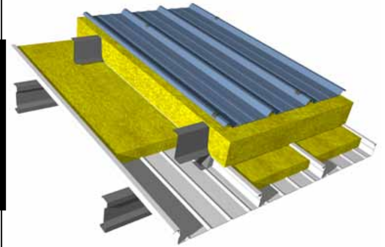
GLOBALROOF IN 226 trames parallèles en couverture / double skin roof
