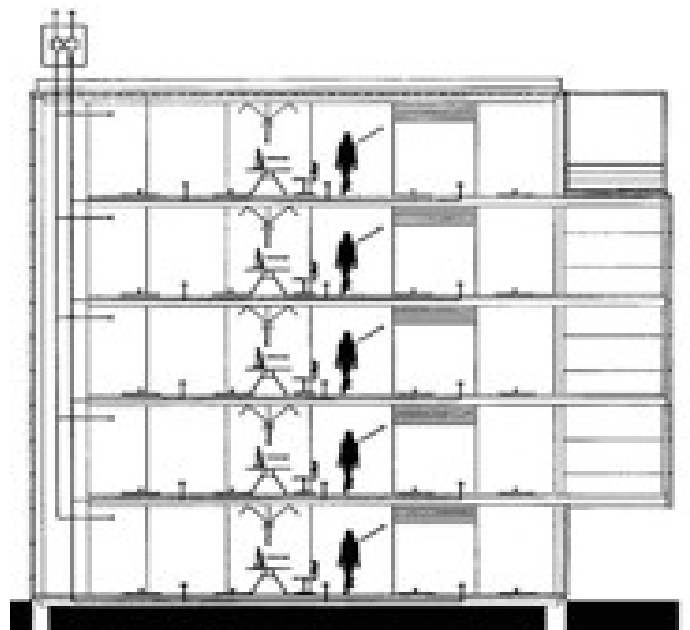
Figure 5 : Bâtiment avec structure légère en acier et planchers « secs »
